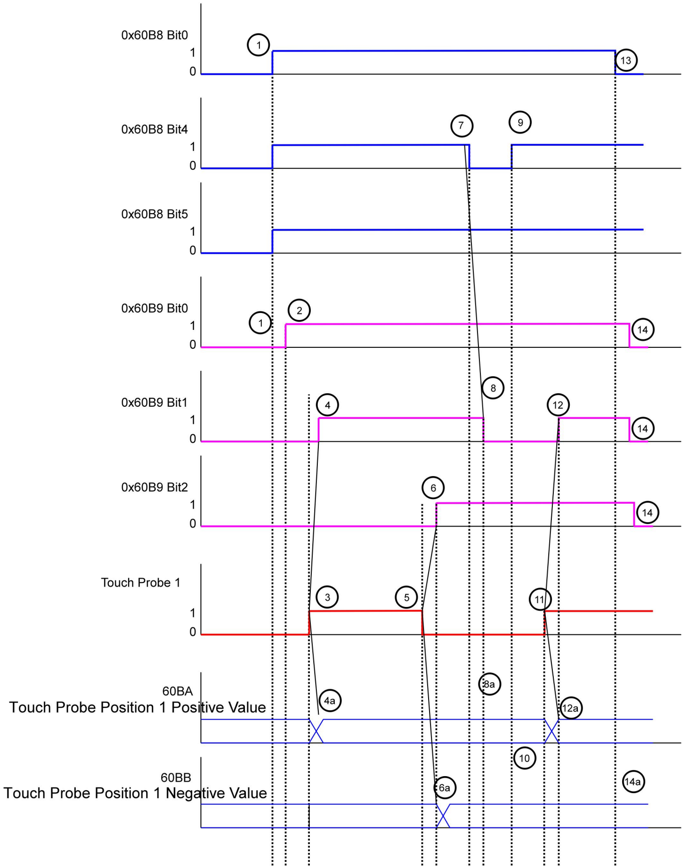
探针时序图
