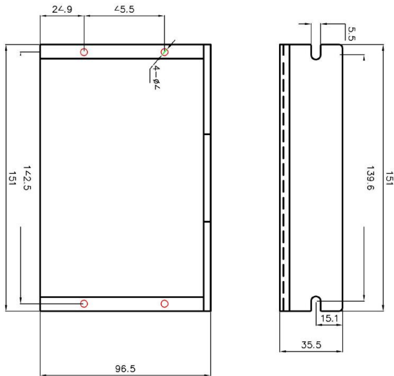
ECR86 安装尺寸
