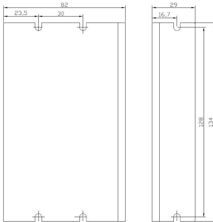
ECR42、5ECR42 安装尺寸
