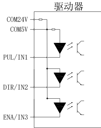
图 3-1 数字输入接口原理
