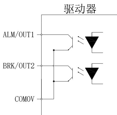
图 5-4 数字输出接口原理
