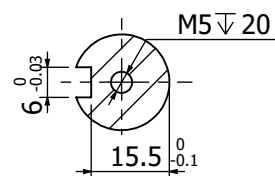
剖面 A-A
