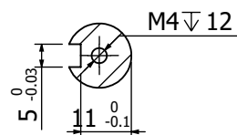
剖面 A-A
