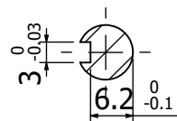
剖面 A-A
