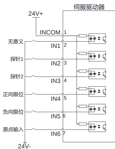
共阳输入
