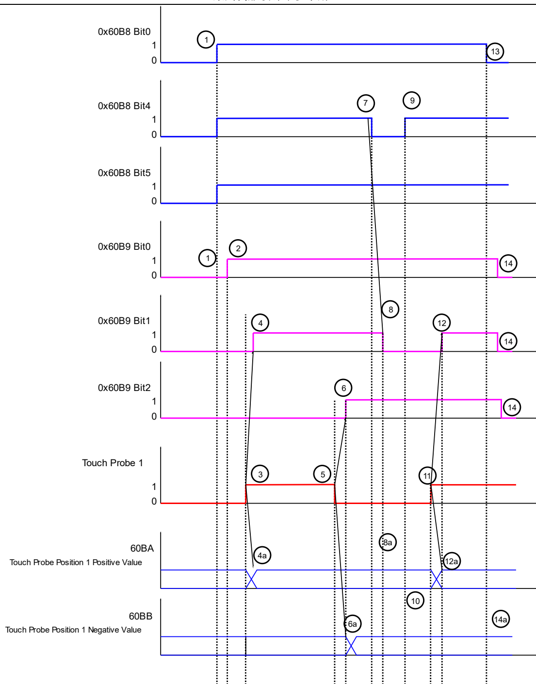
探针时序图
