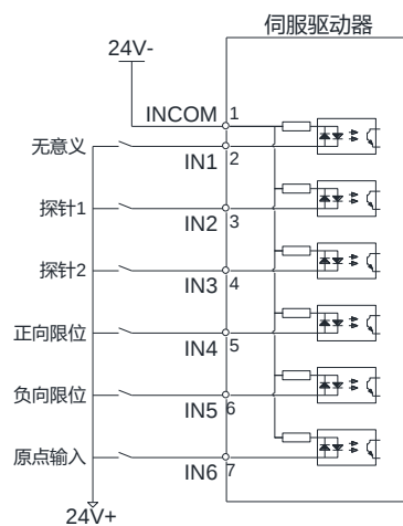
共阴输入
